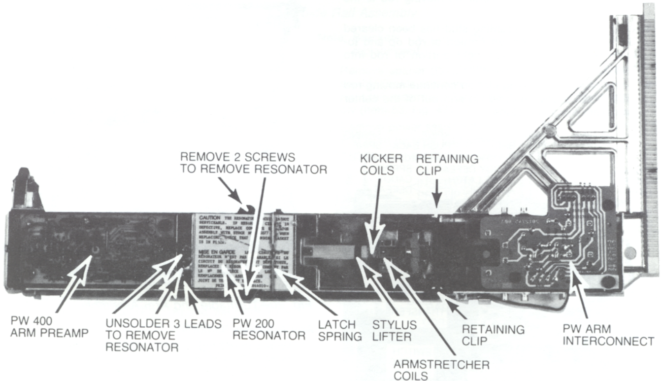
Fig. 21—Arm Assembly
